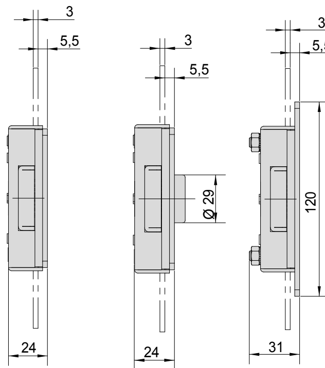
Schloss mit Montagedecken / Lock with mounting covers Z-017 Z-018 / Z-019 Z-032
