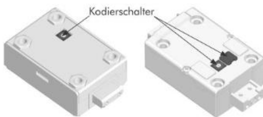
Abbildung 4 - Kodierschalter
