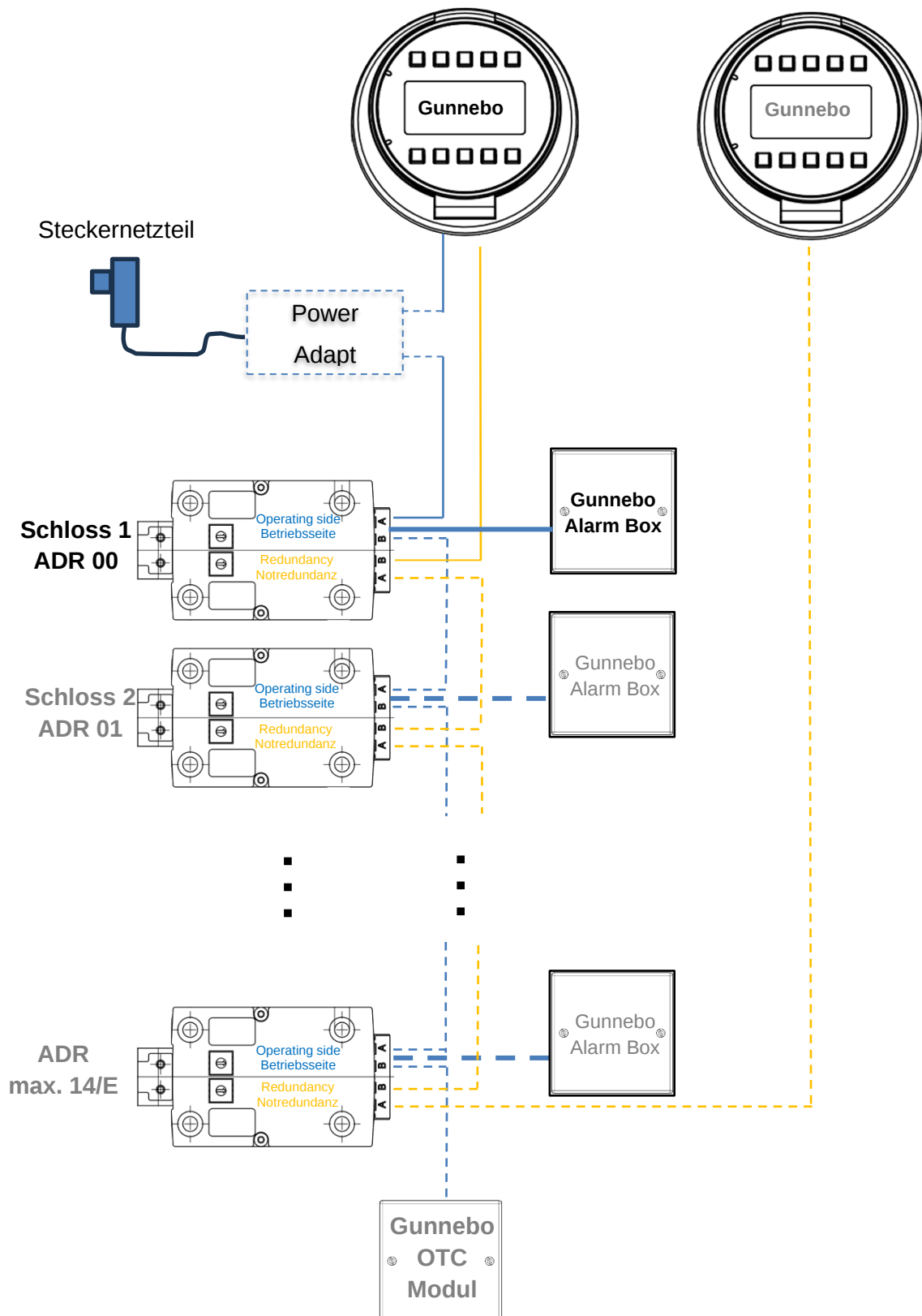
Abbildung 6 - Schaltungstopologie
