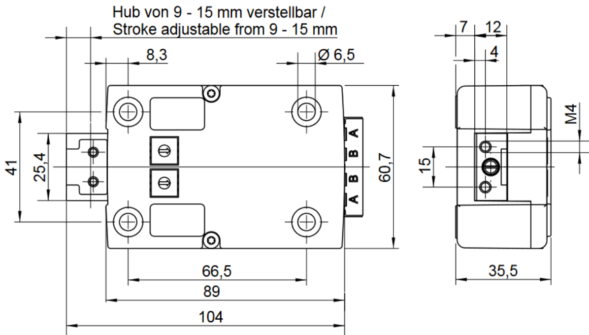
Abbildung 1- Maßzeichnung Gunnebo Encry 600, 800, 900
