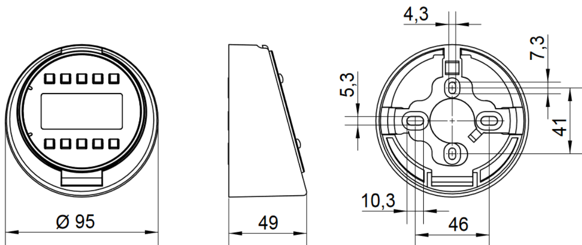
Abbildung 2- Maßzeichnung Tastatur
