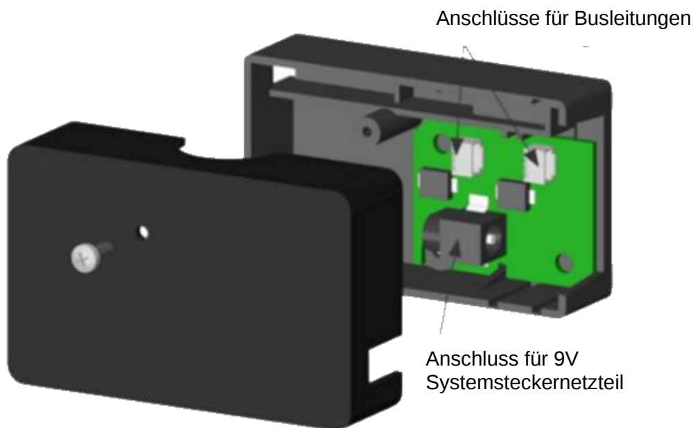
Abbildung 9 - Gunnebo Power Adapt Anschlüsse
