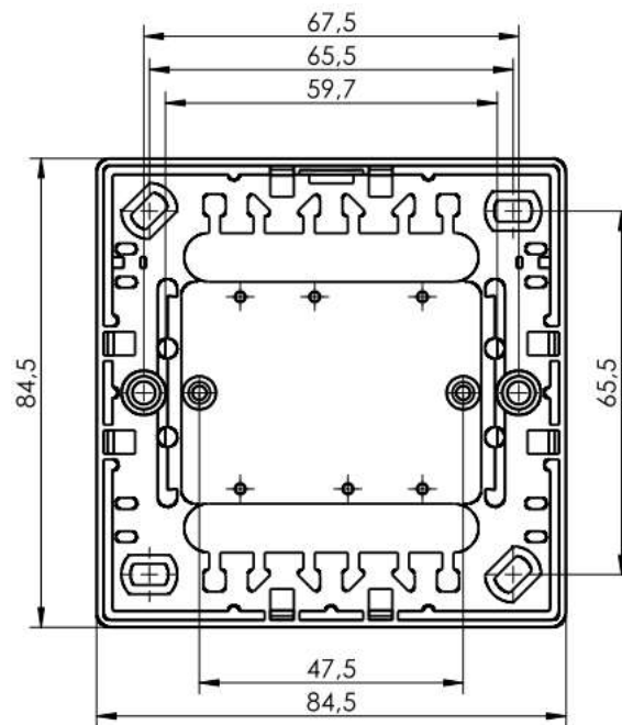
III Gehäusezeichnung
